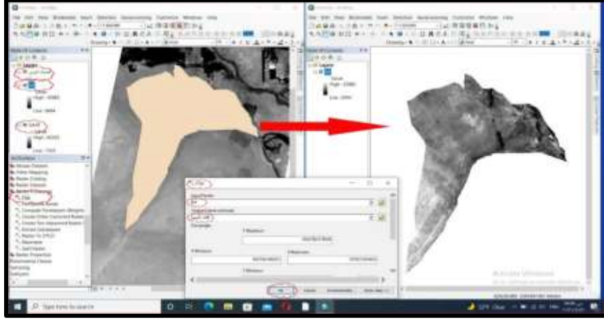
صورة (٢) عملية قطع (Clip) للمرئيات الفضائية لقضاء الزبير
